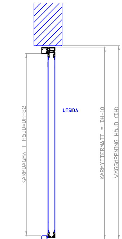
VERTIKALSEKTION
