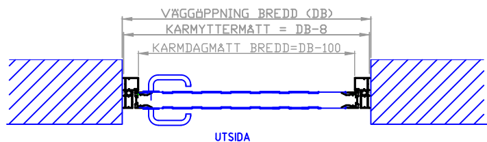
A-A HORIZONTALSEKTION
