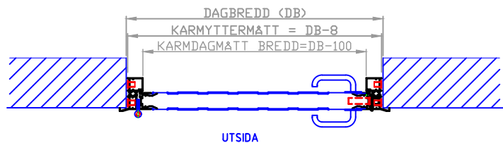
A-A HORIZONTALSEKTION
