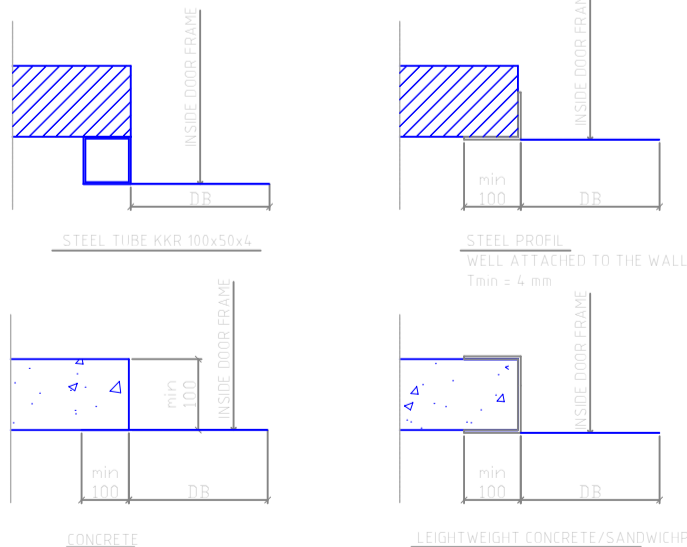
JAMB ALTERNATIVES
