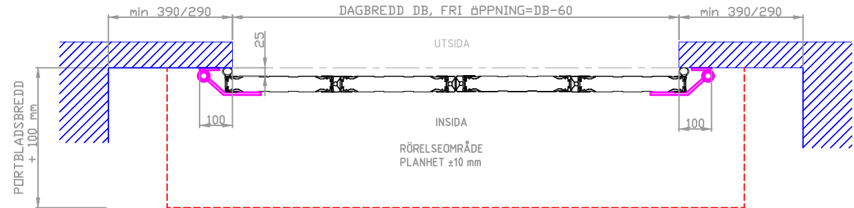
A-A HORIZONTALSEKTION
