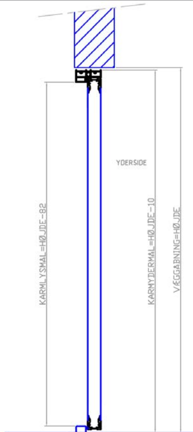
Lodret tværsnit
