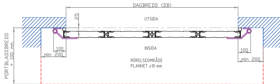
A-A HORIZONTALSEKTION
