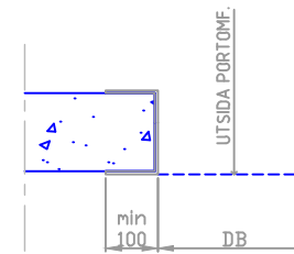
LÄTTBETONG/SANDWICHPANEL U-PROFIL T min = 4 mm 6 mm OM PORTBLAD > 6 kvv
