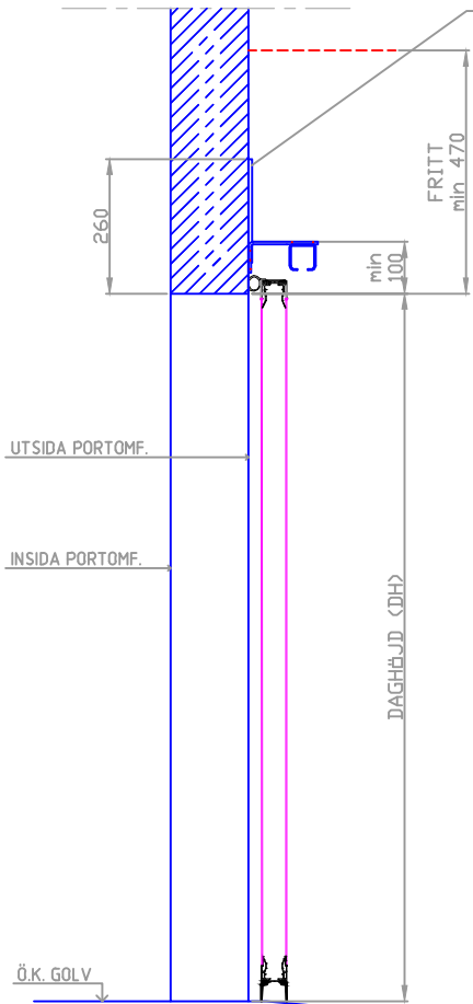
VERTIKALSEKTION
