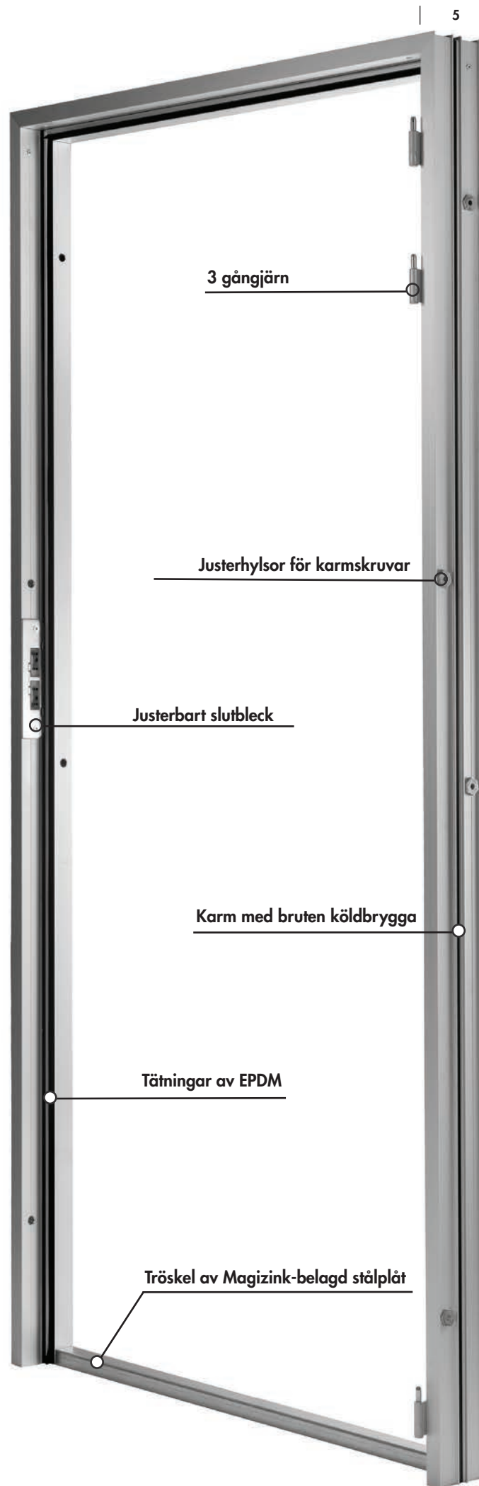
Karm med bruten köldbrygga
