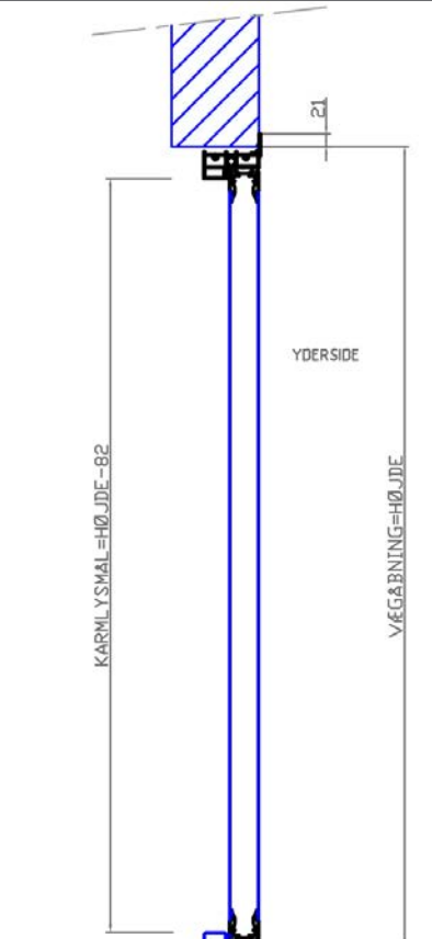
Lodret tværsnit
