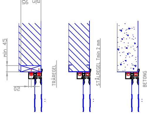
VERTIKALSEKTION
